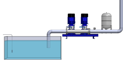
Basınç Anahtarı ile Kontrol
