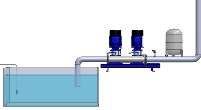
Basınç Sensörü ile Kontrol
