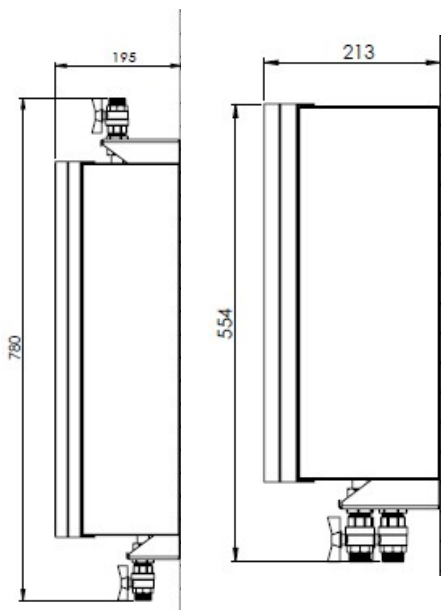
Duvara Montaj Görünüşü
