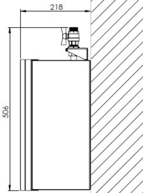
Duvara Montaj Görünüşü
