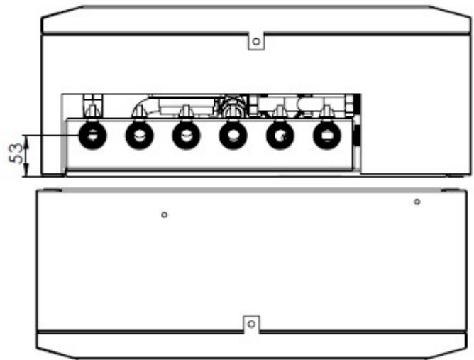
Alt Görünüş
