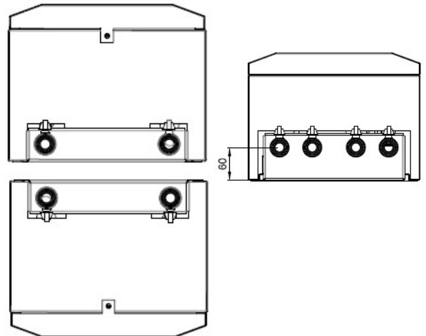
Alt Görünüşü
