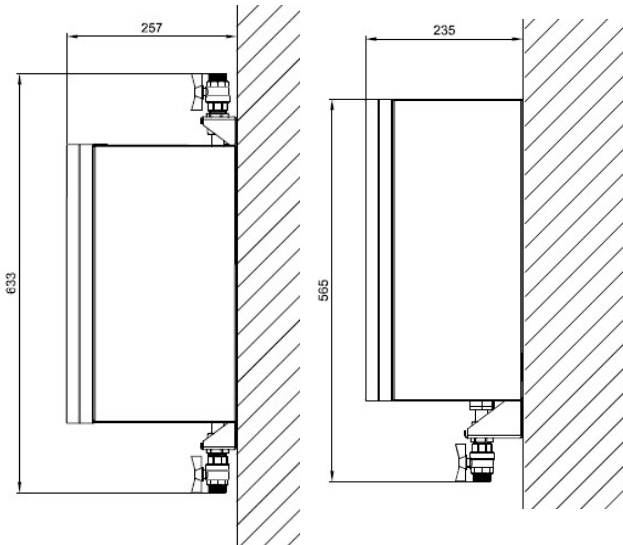
Duvara Montaj Görünüşü
