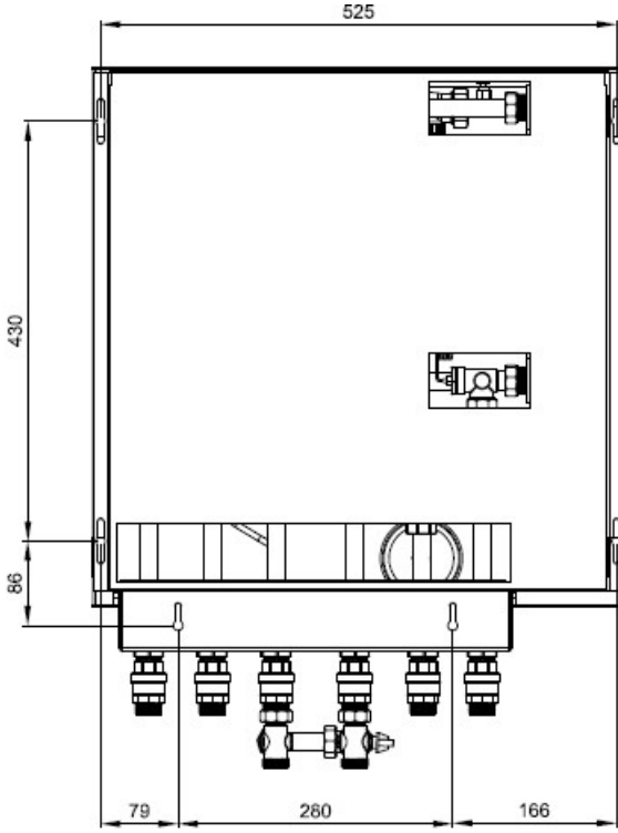
Duvara Montaj Görünüşü
