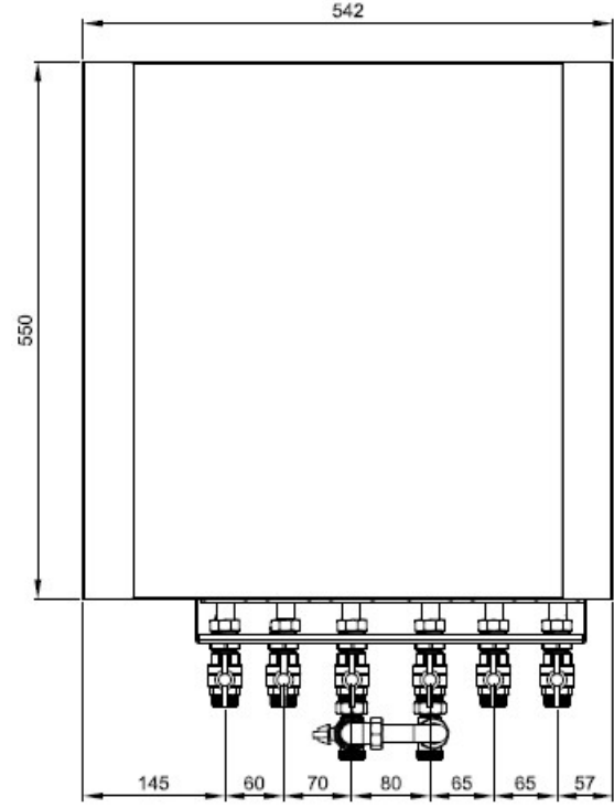
Alt Görünüş
