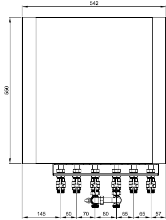
Önden Görünüm
