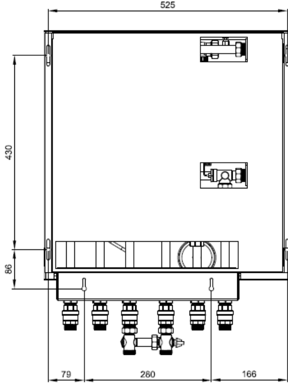
Arka Görünüm
