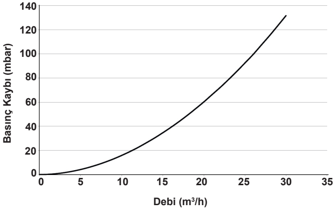
DN50 Basınç Kaybı Eğrisi
