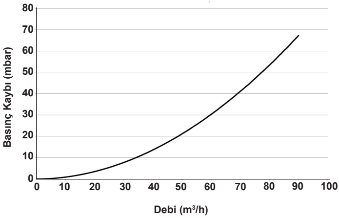
DN200 Basınç Kaybı Eğrisi
