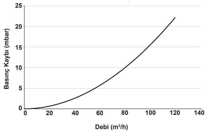
DN150 Basınç Kaybı Eğrisi
