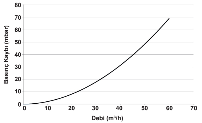
DN80 Basınç Kaybı Eğrisi
