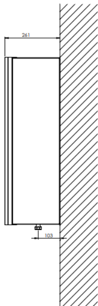
Duvara Montaj Görünüşü
