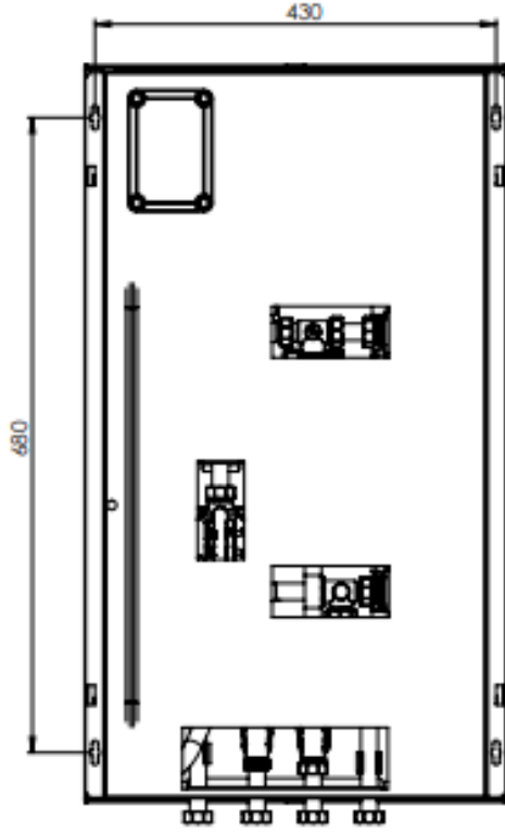
Duvara Montaj Görünüşü
